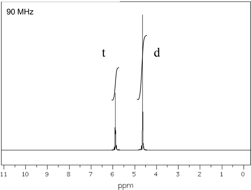
^1\text{H} NMR
