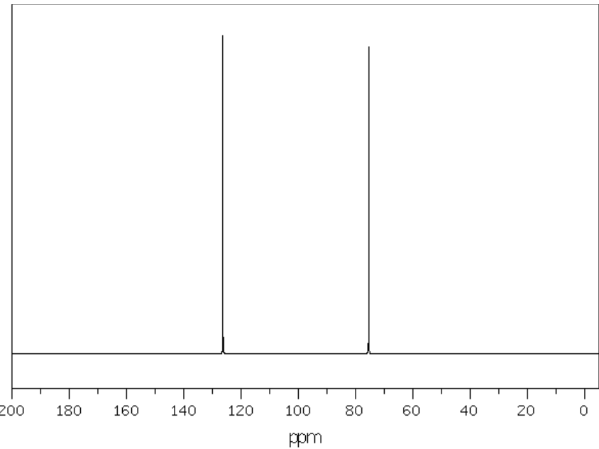
^{13}\text{C} NMR
