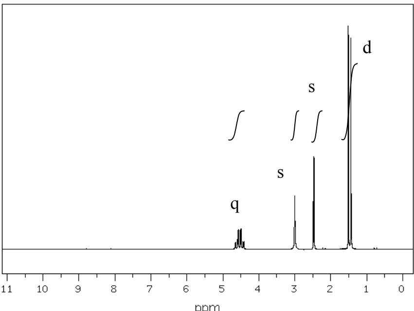
1 H NMR
