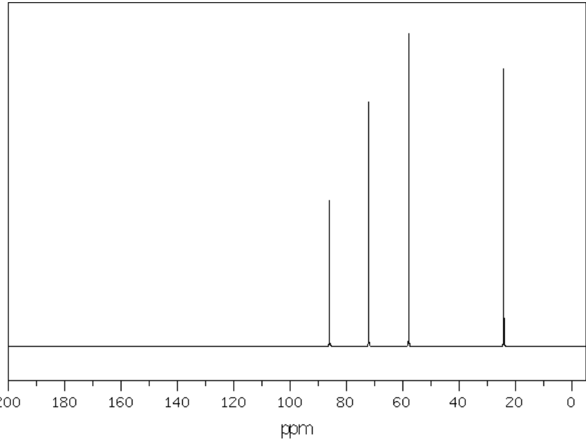
13 C NMR
