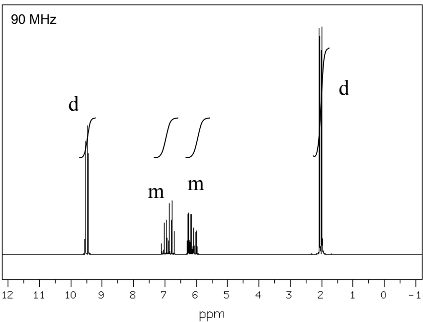
^1\text{H} NMR
