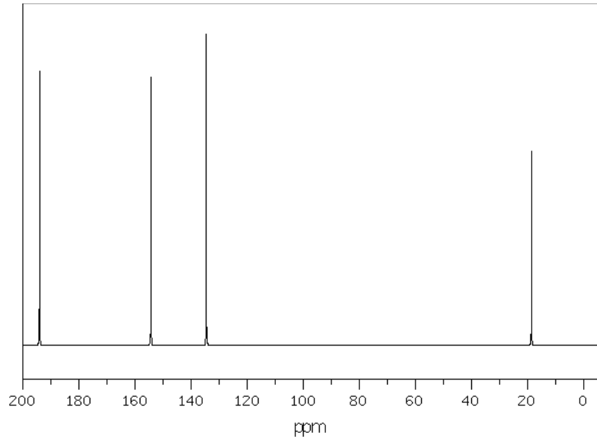
^{13}\text{C} NMR
